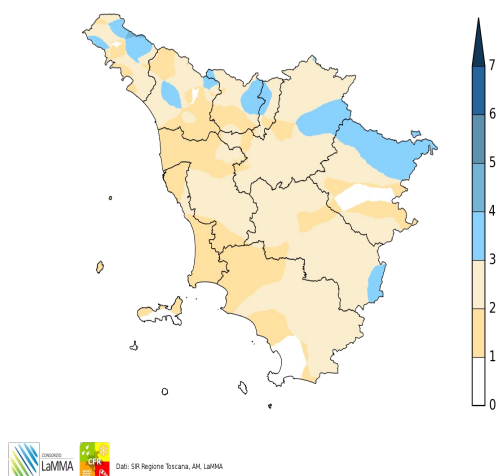
Giorni con Pioggia \geq di 0.4 mm dal 12/07/2018 al 18/07/2018
