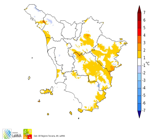
Anomalia Temperatura Minima settimanale dal 12/07/2018 al 18/07/2018
