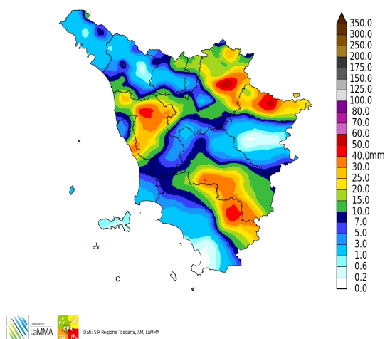
Cumulato Precipitazione dal 12/07/2018 al 18/07/2018
